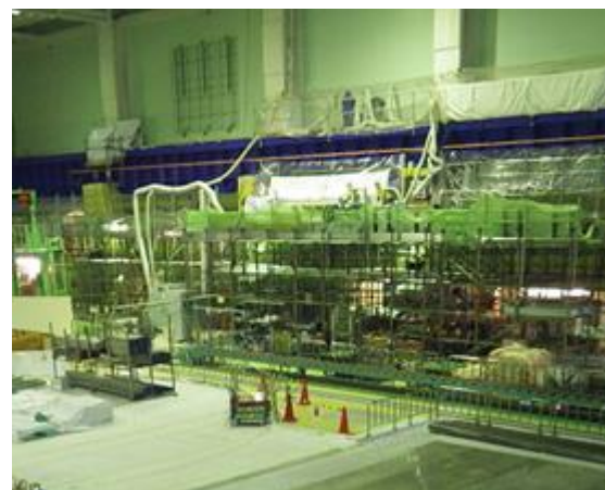
原子炉建屋最上階 工事中の状況
